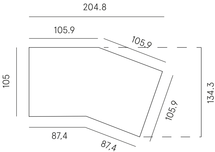
Modulo Angolo
