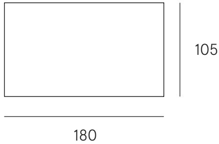
Modulo/Module 180 cm
